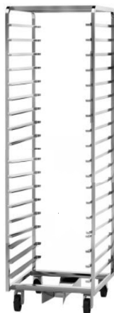
ТЕЛЕЖКА ДЛЯ РОТАЦИОННОЙ ПЕЧИ MACADAMS (МАКАДАМС) МОДЕЛЬ М 60; М100 ; М179 505Х810Х1800, 12 ПРОТИВНЕЙ НЕРЖАВЕЮЩАЯ СТАЛЬ
