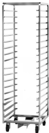
ТЕЛЕЖКА ДЛЯ РОТАЦИОННОЙ ПЕЧИ MACADAMS (МАКАДАМС) МОДЕЛЬ М 60; М100 ; М180 505Х810Х1800, 16 ПРОТИВНЕЙ НЕРЖАВЕЮЩАЯ СТАЛЬ
